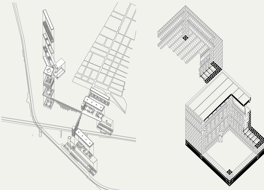
Axonométrie de projet Axonométrie constructive
