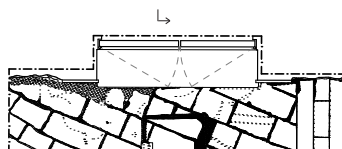
DETAGLIO ARCHITETTONICO 3 SCALA 1:20
