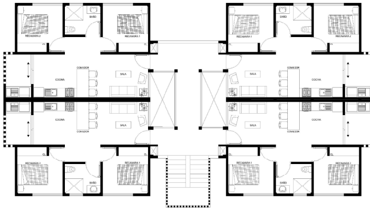
PLANTA ARQUITECTONICA TIPO 3° Y 4° NIVEL
