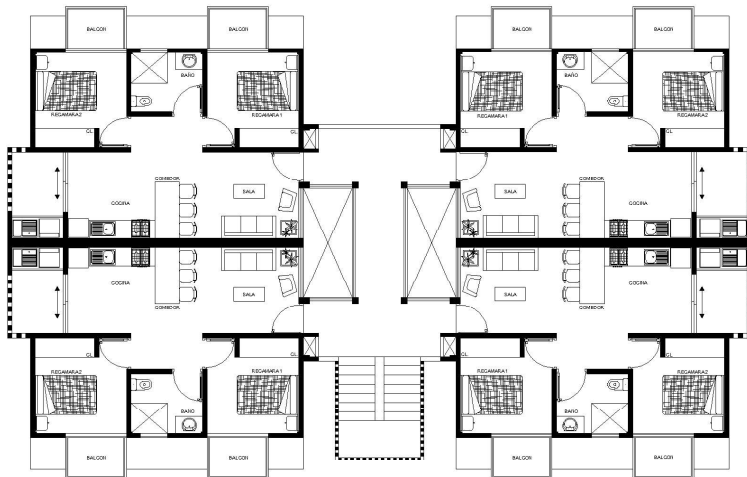
PLANTA ARQUITECTONICA 2° NIVEL
