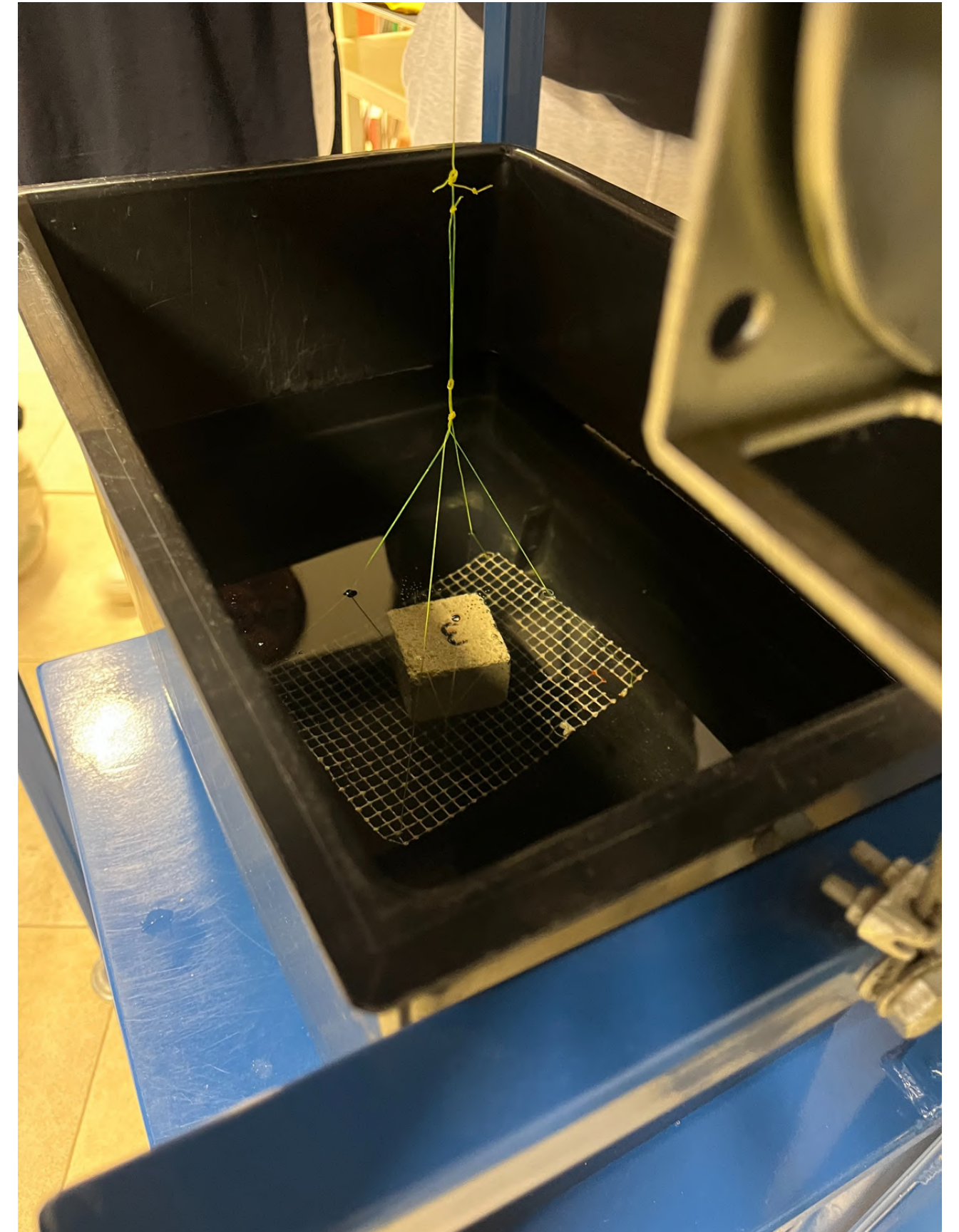
Photographie d'un échantillon de béton ; poids du volume submergé
