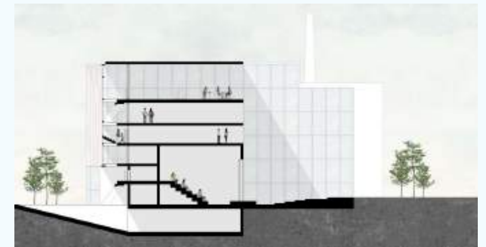
Coupe-élévation
