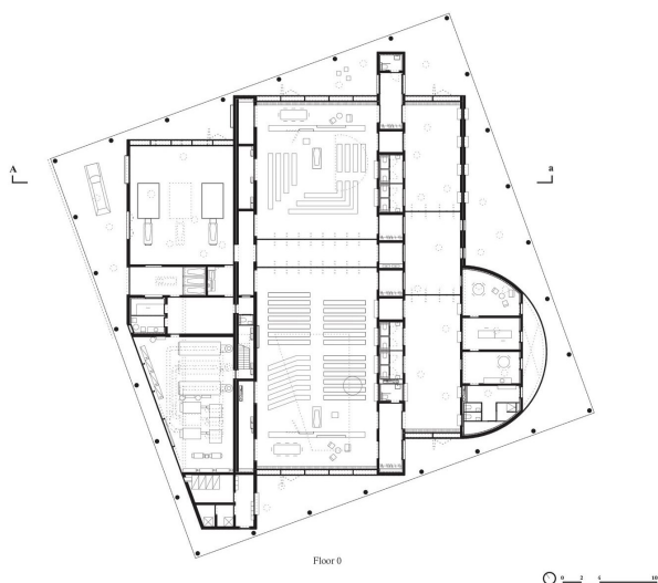
Fig. 7 OFFICE Kersten Geers David Van Severen, Crematorium Ostende - 2014
