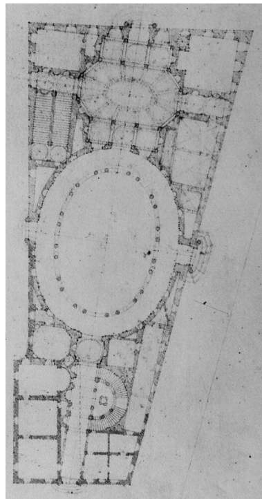
Fig. 6 Borromini Palais Carpegna, Rome, 1647
