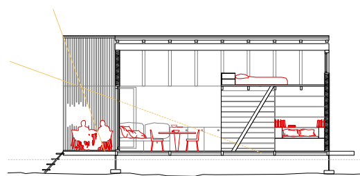
Coupe longitudinale
