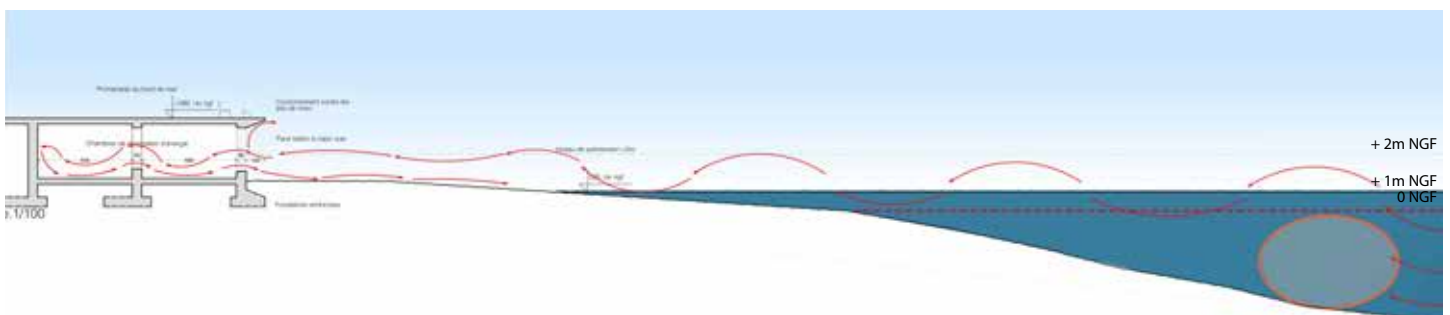
Configuration projetée : principe de mur caissons à dissipation d'énergie
