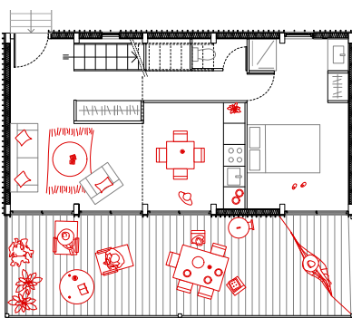
Plan rez-de-chaussée
