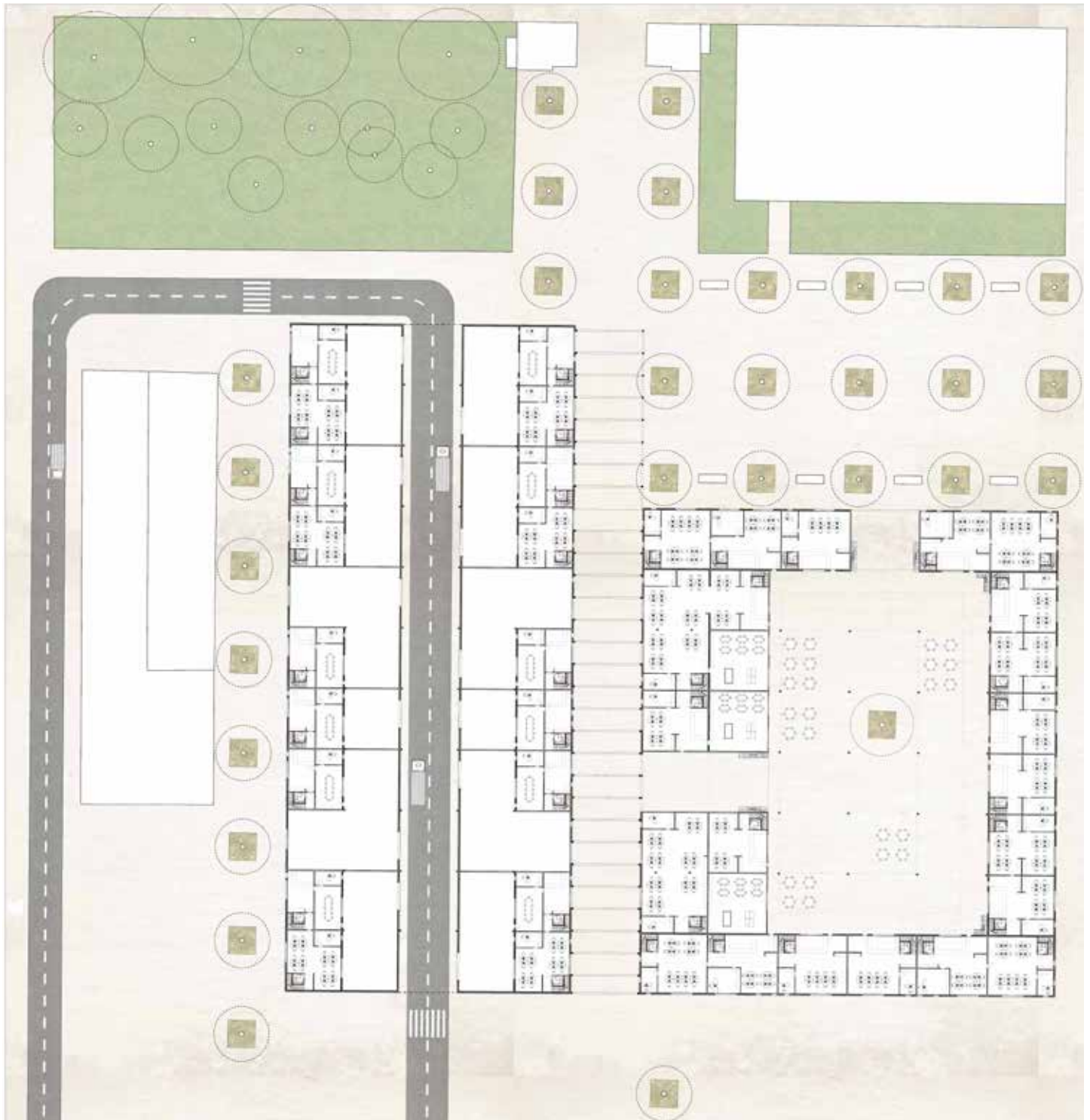
Plan de rez-de-chaussée
